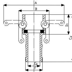
TÖMLŐCSONKOS ANYA C TÍPUS
