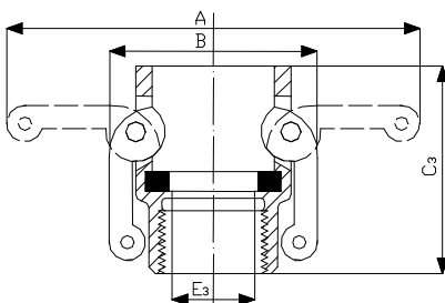
MENETES ANYA D TÍPUS
