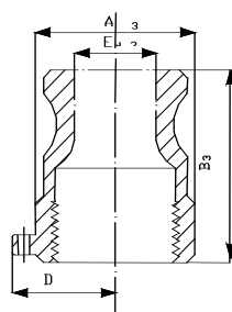
MENETES APA A TÍPUS
