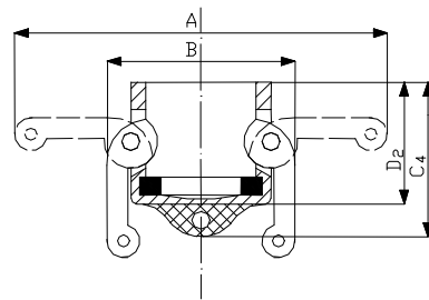
ZÁRÓANYA DC TÍPUS
